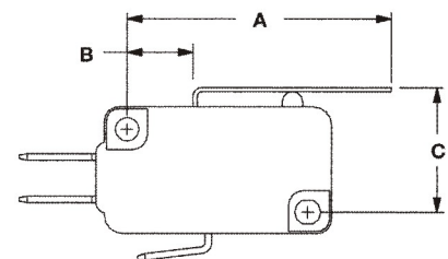
FIG. 3 Lever
