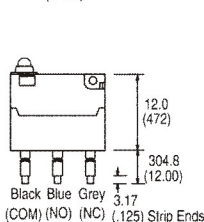
J WIRE LEADS BOTTOM (IP67)
